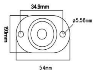
HW1962 Terminal Stud 3/8"-16 Black
