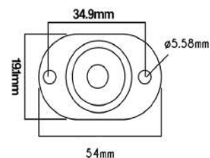
HW1406 Terminal Stud 3/8"-16 Red
